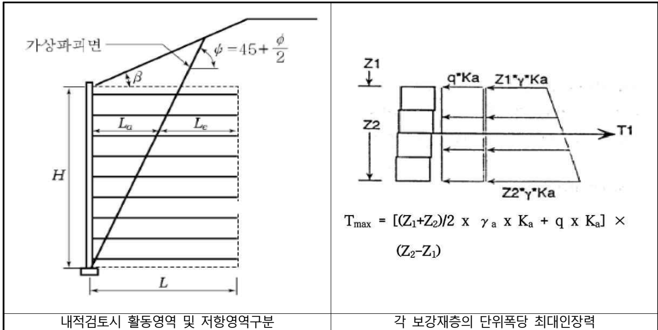
토압작용 모식도
